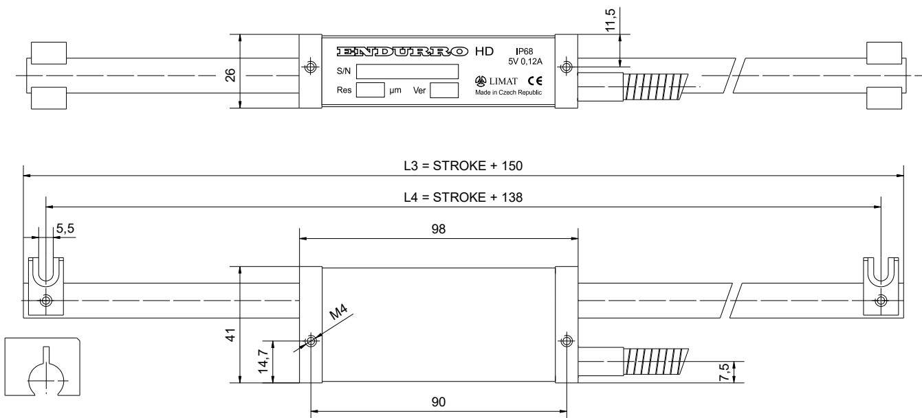
Snímač s pevnými příchytkami Sensor with fix clips
